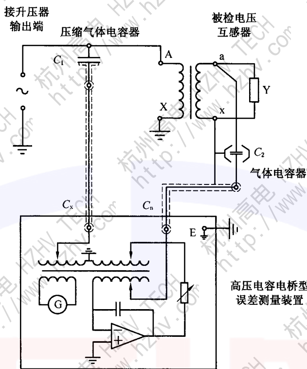
(b) 使用高压电容电桥型误差测量装置的检定线路
