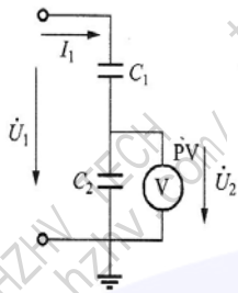
图3 电容分压器与低压电压表组成测量系统的原理接线图
