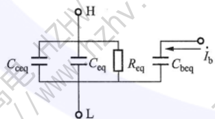
图 A.2 高压电容的等效电路
