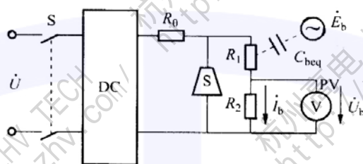
图 A.1 测量带电导体与电阻分压器之间耦合电容电流 I_b 的原理接线
