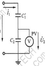
图 A.4 电容分压器计算用等效电路图
