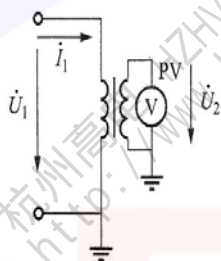
图 5 高压电压互感器与低压电压表组成的测量系统的原理接线图
