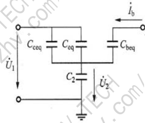
图 A.5 考虑带电导体影响的电容分压器的等效电路图
