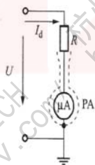
图1 高阻值电阻器与直流微安表串联的测量系统的原理接线图
