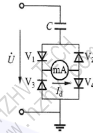
图4 高压电容器与整流桥串联的测量系统的原理接线图
