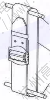
图 A.3 登杆脚扣扣带强力试验试样装夹方法示意图
