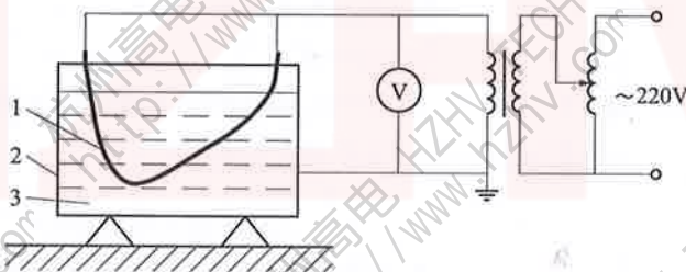
图 B.2 核相器连接导线绝缘强度试验接线图
