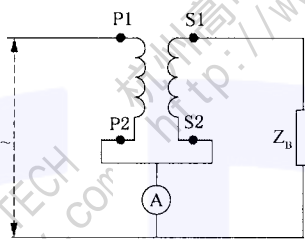
图 2D.4 1 : 1 电流互感器的基本电路
