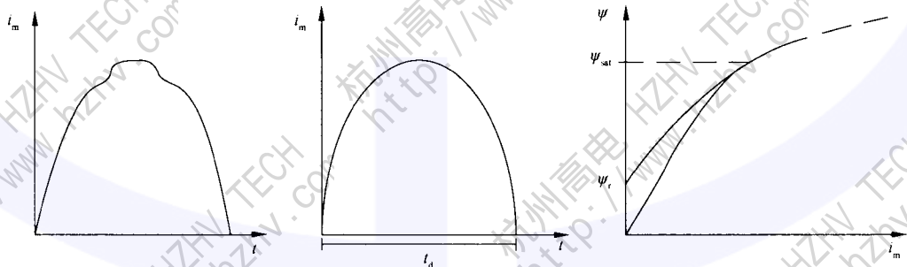
图 2E.14 电容放电法的典型记录图
