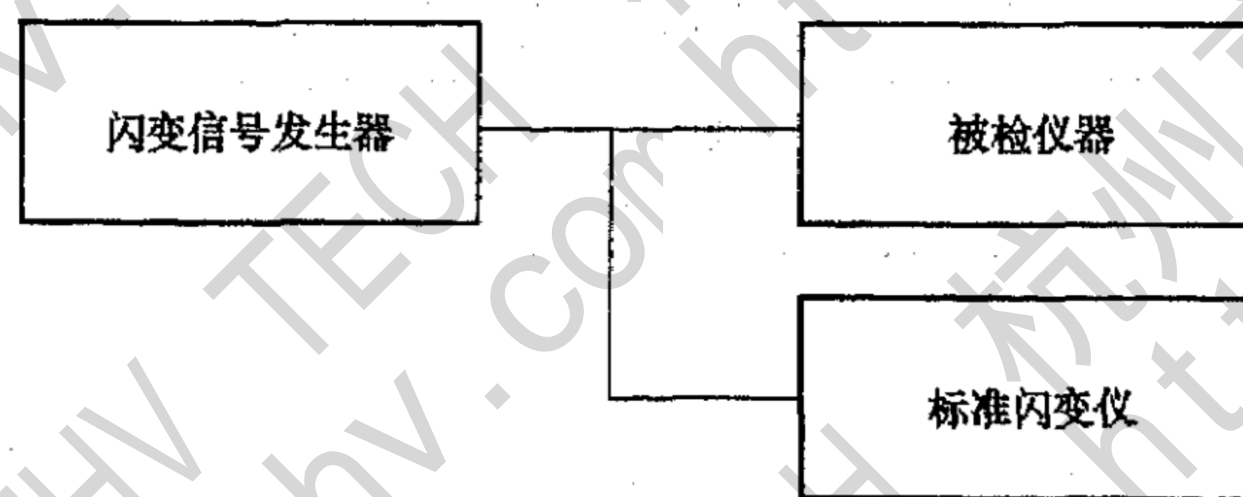
图 10 标准仪器法闪变值检定示意图
