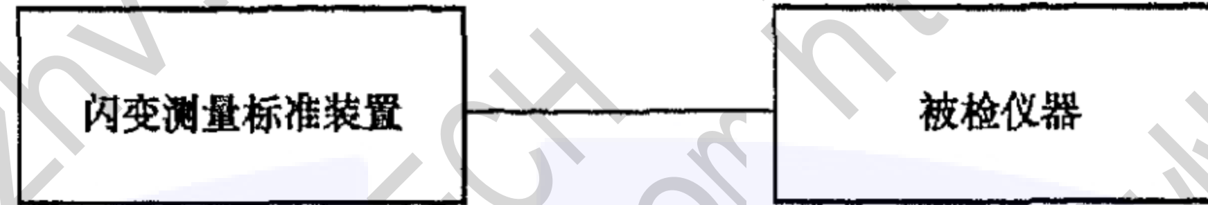
图 9 标准源法闪变值检定示意图
