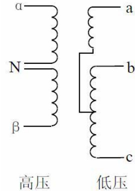
逆斯科特变压器原理图
