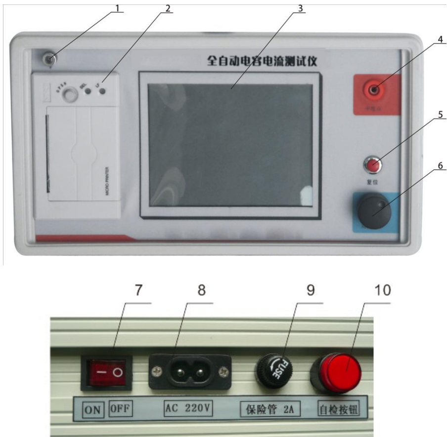
图 1 仪器外观
