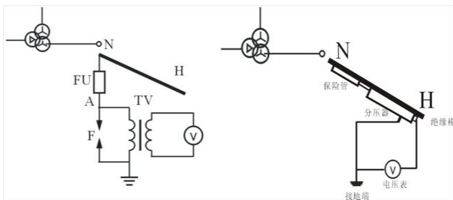
图 10a 用 PT 测量中性点电压
