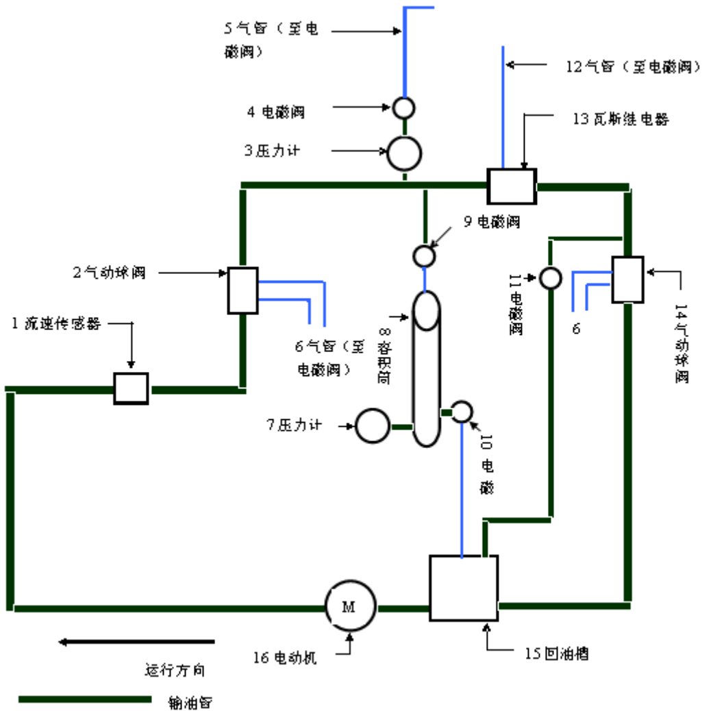
图二油路图
