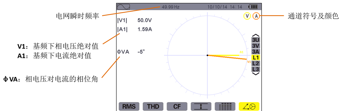
图 8-21 L1 下矢量图显示屏
