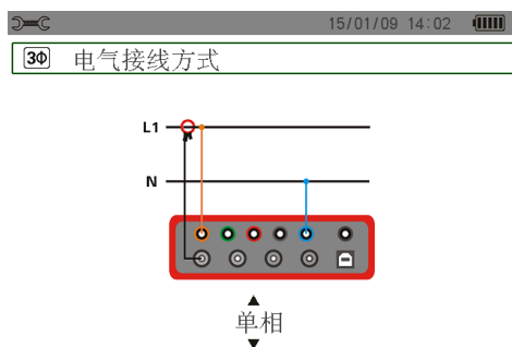
图 4-4 单相连接
