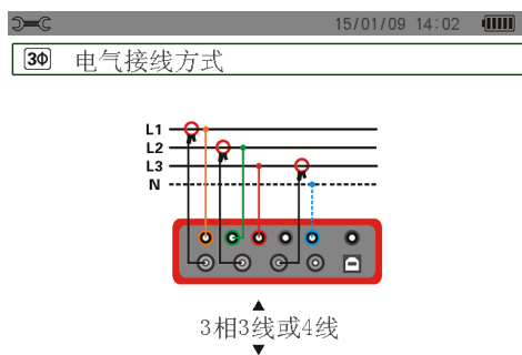
图 4-6 三相 3 线或 4 线连接
