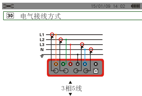
图 4-7 三相 5 线连接
