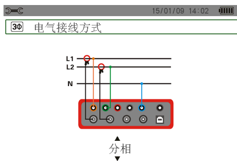
图 4-5 分相连接
