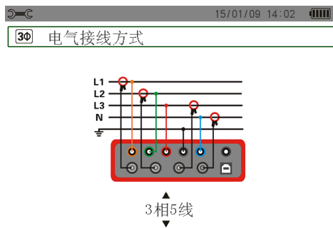
图 5-6 电气连接方式选择
