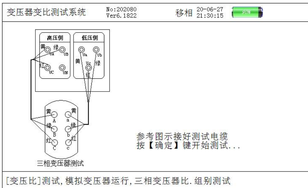
图五、三相变比测试接线提示屏
