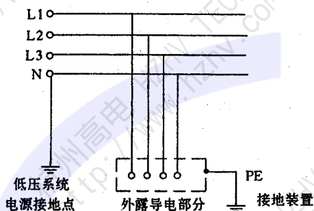
图 4 TT 系统
