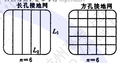
图 B1 接地网的形状
