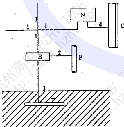
图 6 建筑物内总等电位联结图
