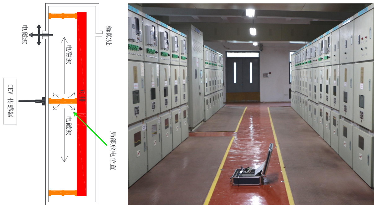
图 3-1 TEV 检测原理图
